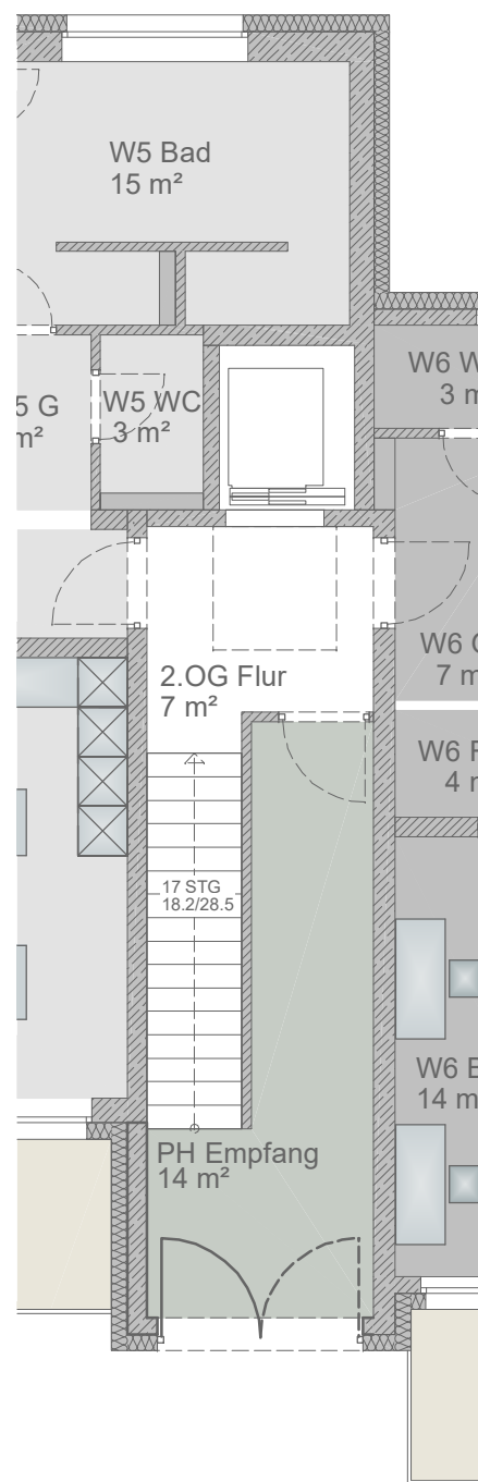
Grundriss 2.OG
