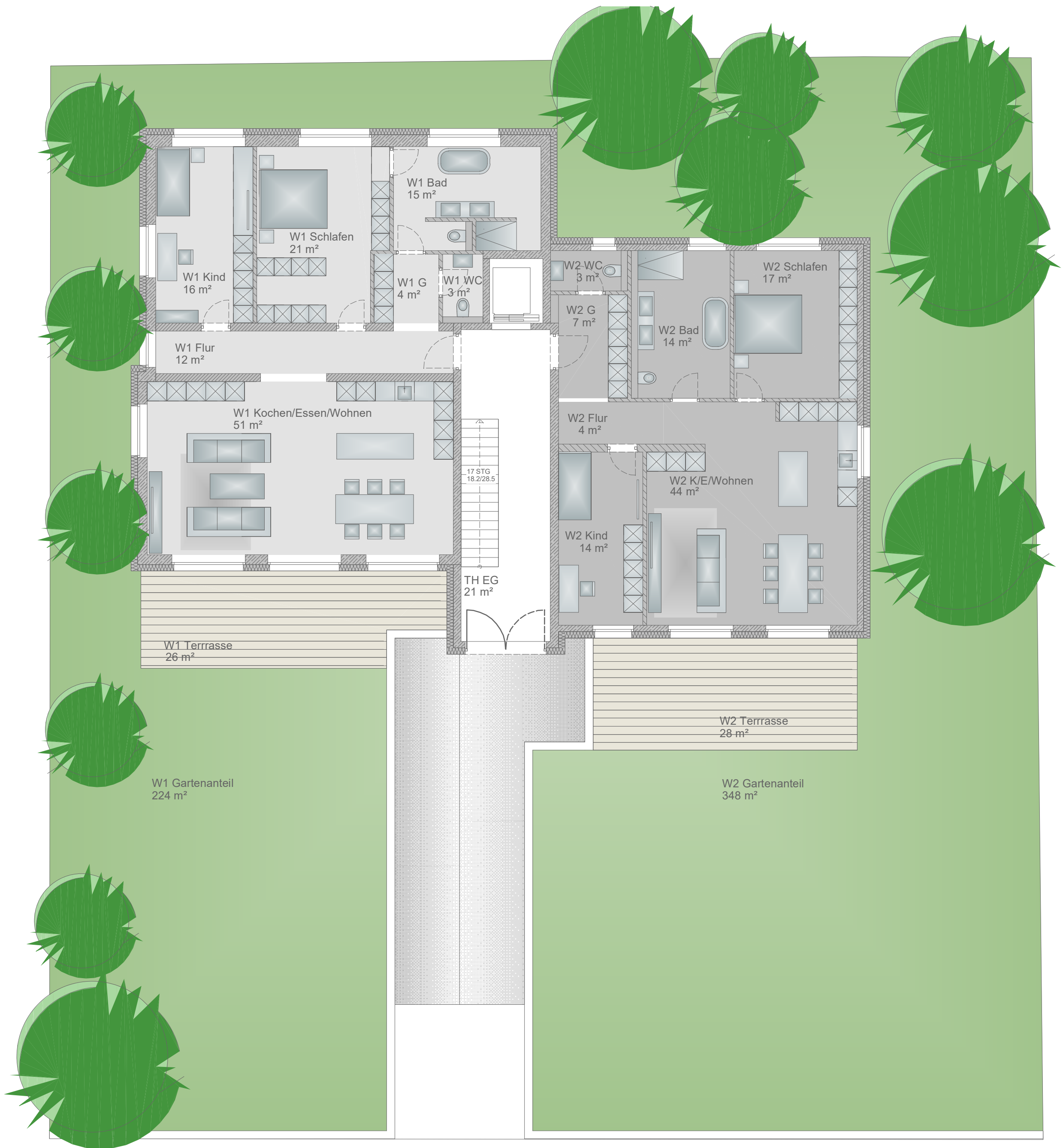
Grundriss EG
